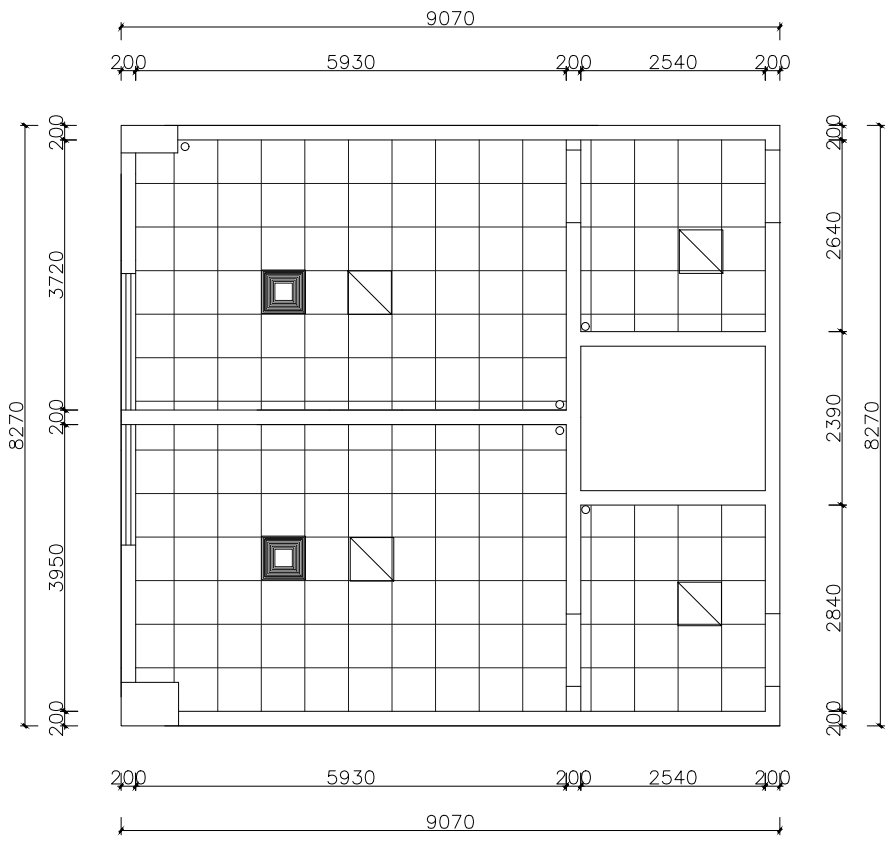
天花吊顶图
