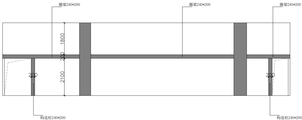
砌墙梁柱构造图
